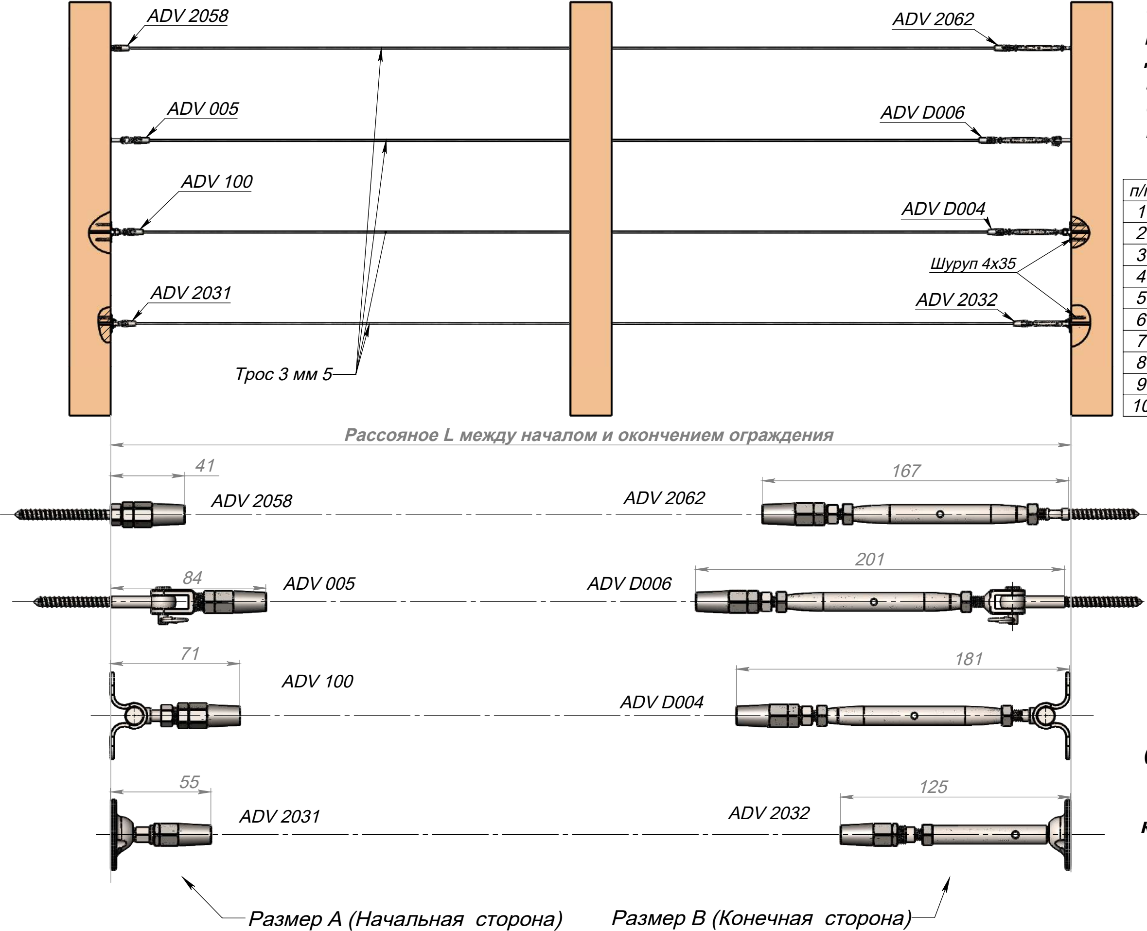
Схема 2 рекомендуемых вариантов установки системы тросов с использованием цанговых наконечников
